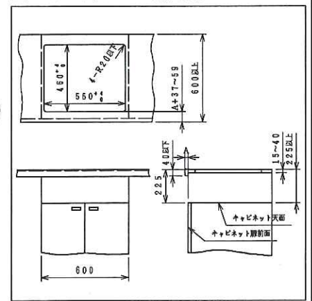
■システムキッチンとの関係寸法
